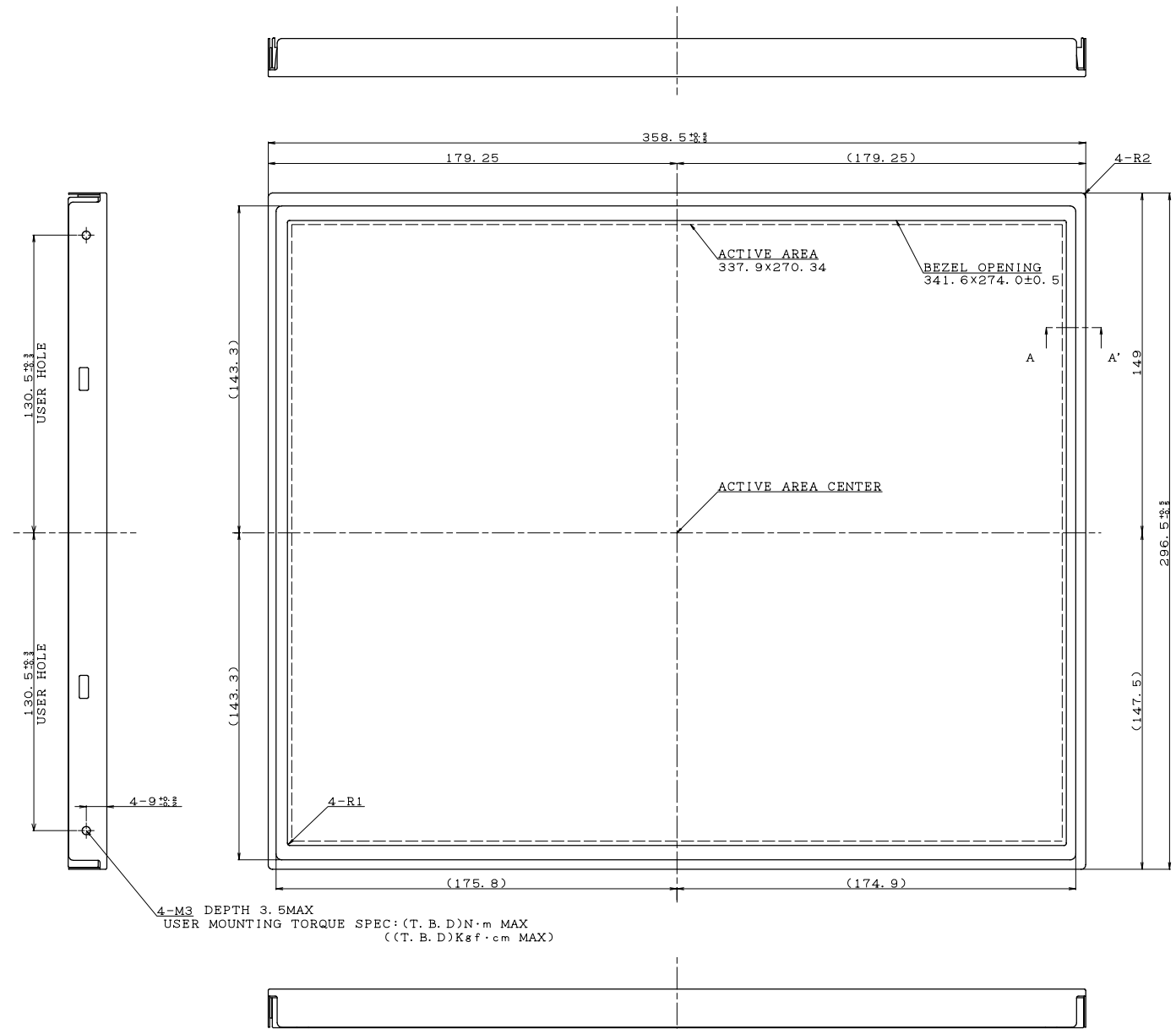
LQ170E1LG11 OUTLINE DIMENSIONS
